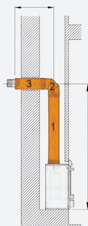
VUE COTÉ Ventouse horizontale standard (pièces 1, 2, 3)
