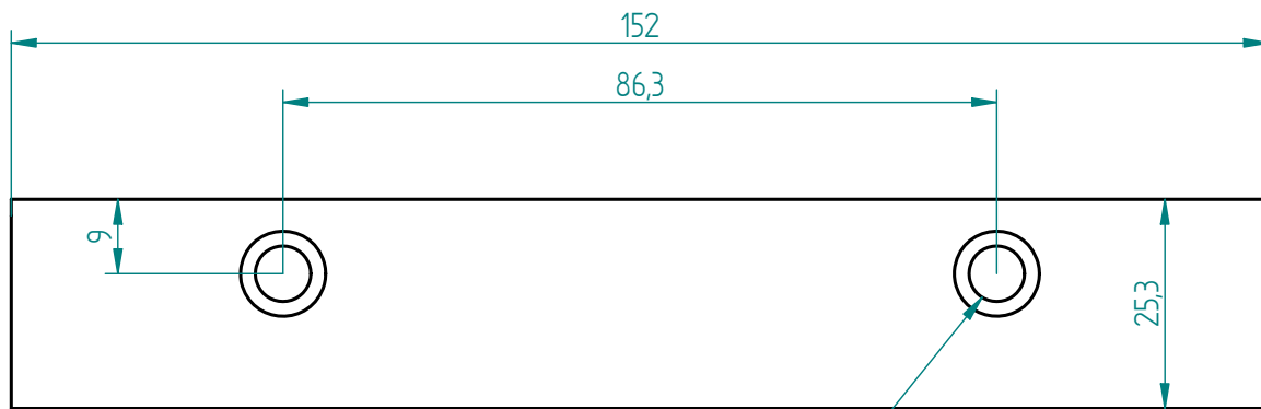
MORDAZA ACERO 150
