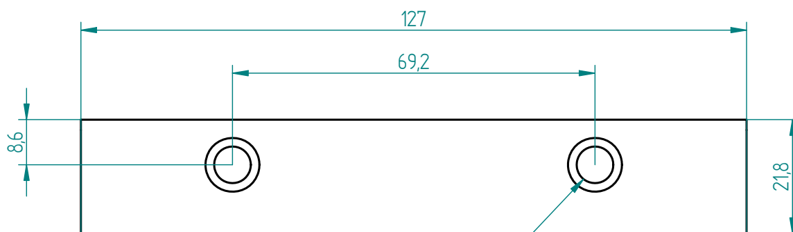
MORDAZA ACERO 125
